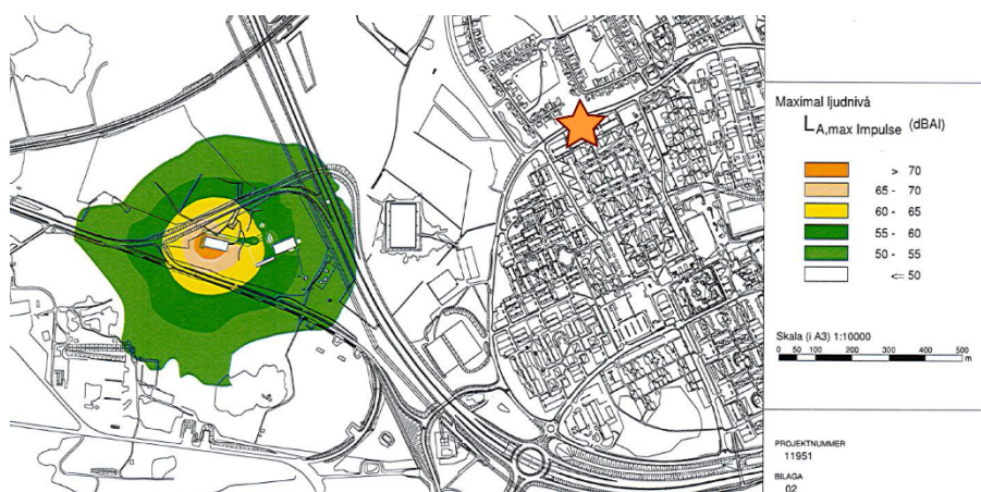
Kartering av maximal ljudnivå dBA, vid skjutning med pistol. Planområdet markerat med en stjärna.
