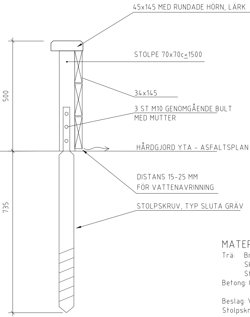
SARG/RINK FÖR BOLLPLAN SEKTION, SKALA 1:10
